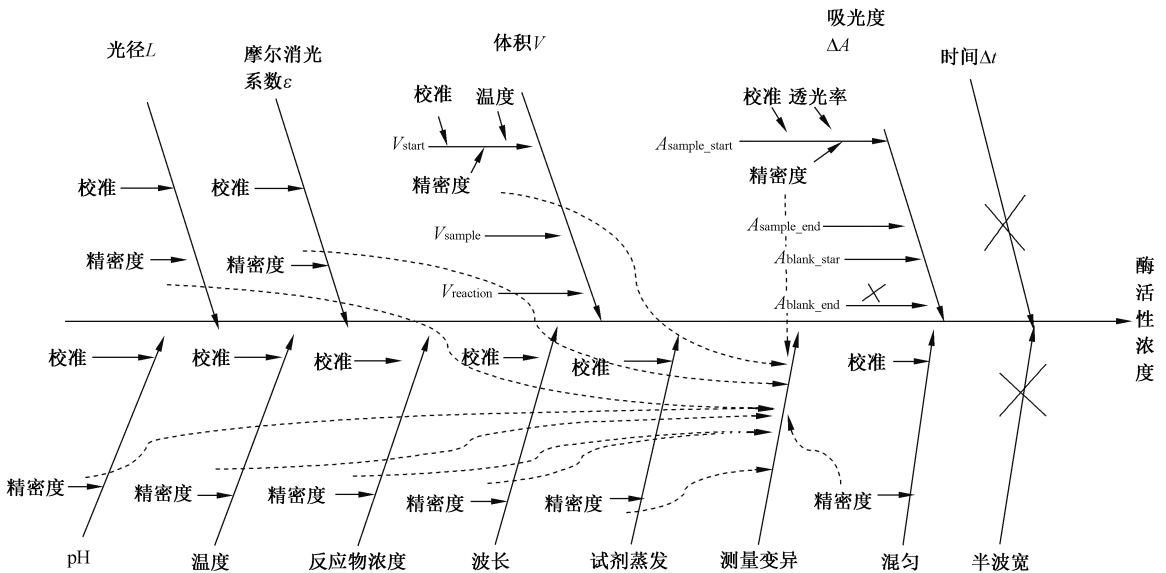
图 4 修正因果图
