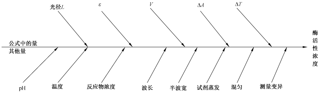
图 3 初步因果图
